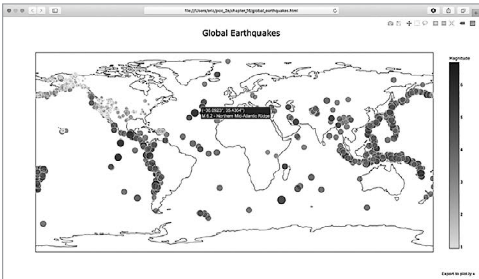
Рис. 16.9. Цвета и размеры маркеров представляют магнитуду землетрясений
