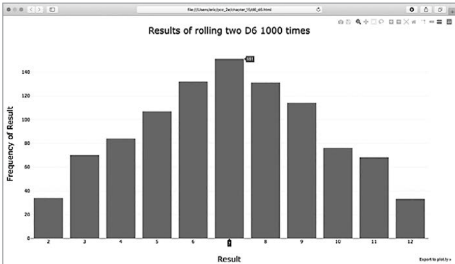
Рис. 15.13. Смоделированные результаты 1000 бросков двух шестигранных кубиков
