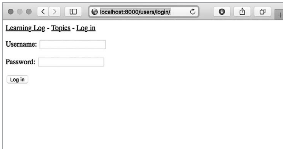
Рис. 19.4. Страница входа
