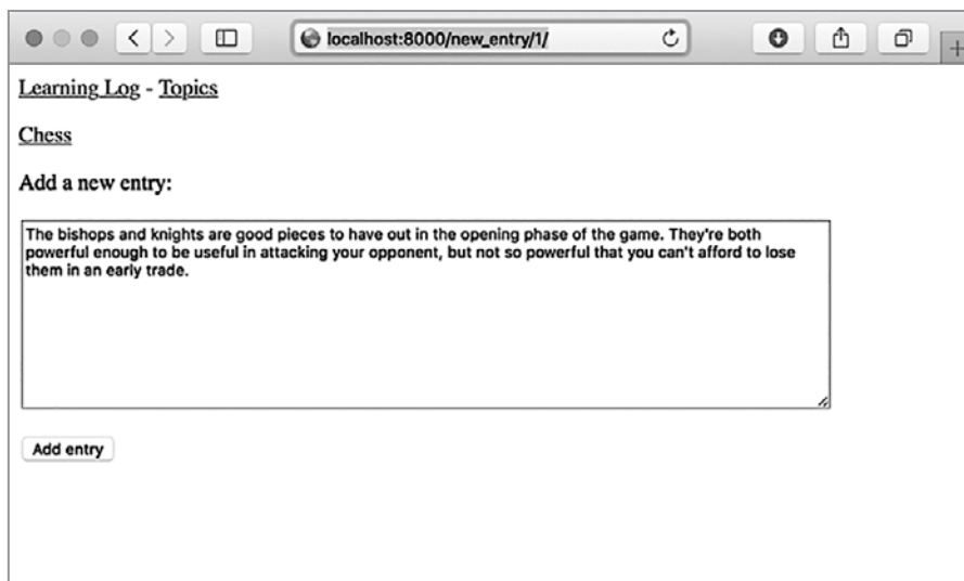
Рис. 19.2. Страница new_entry
